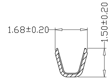
SEC:B-B
